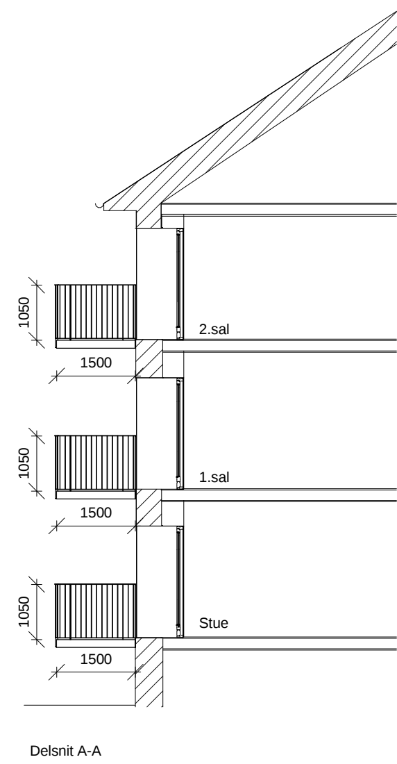
Delsnit A-A
